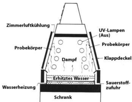
Abbildung: Vereinfachter schematischer Aufbau eines QUV-Schnellbewitterungsgerätes, Quelle: (Q-Panel Company)
